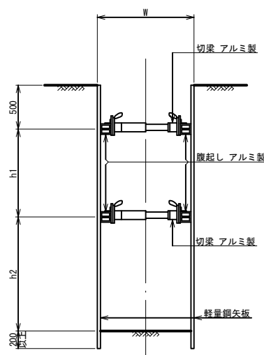
二段支保断面図 (2.0m < 掘削深 ≤ 3.5m)
