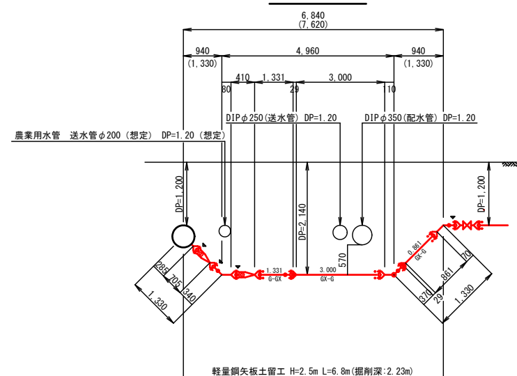
断面詳細図(2)
