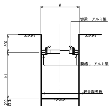
一段支保断面図 (掘削深 ≤ 2.0m)
