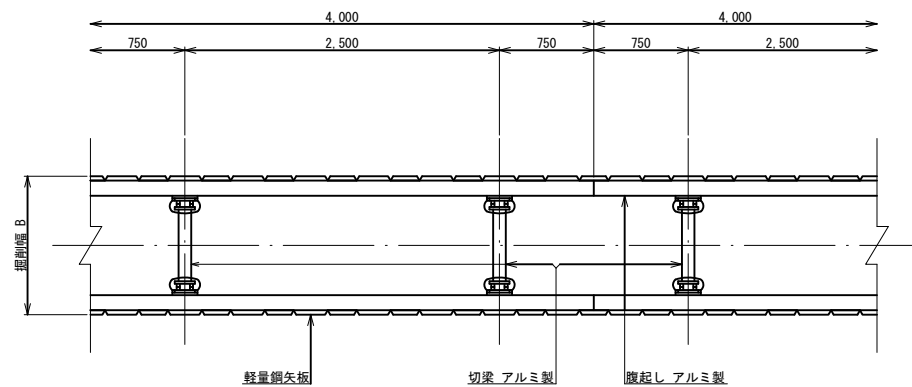
一段支保断面図 (掘削深 ≤ 2.0m)
