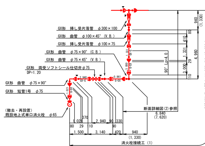
消火栓接続工(1)
