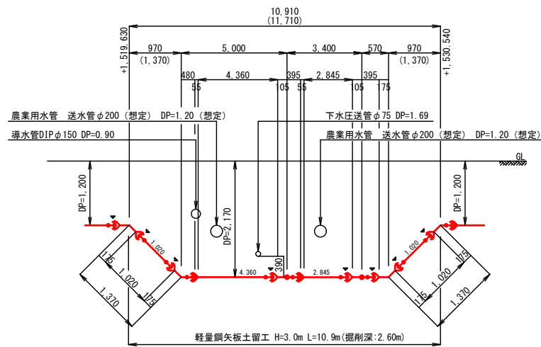
断面詳細図(1)
